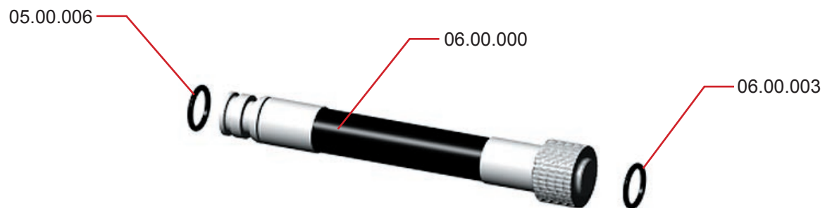
Шланг АИР-98МИ.06.00.000
