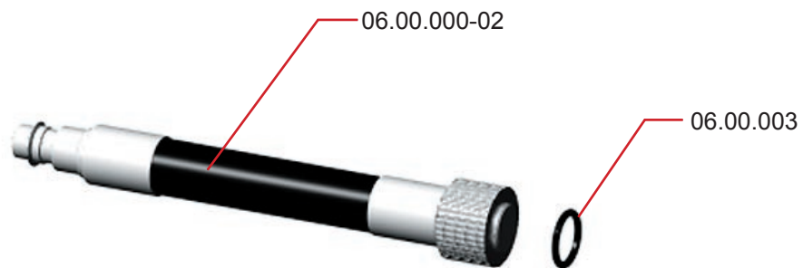
Шланг АИР-98МИ.06.00.000-02
